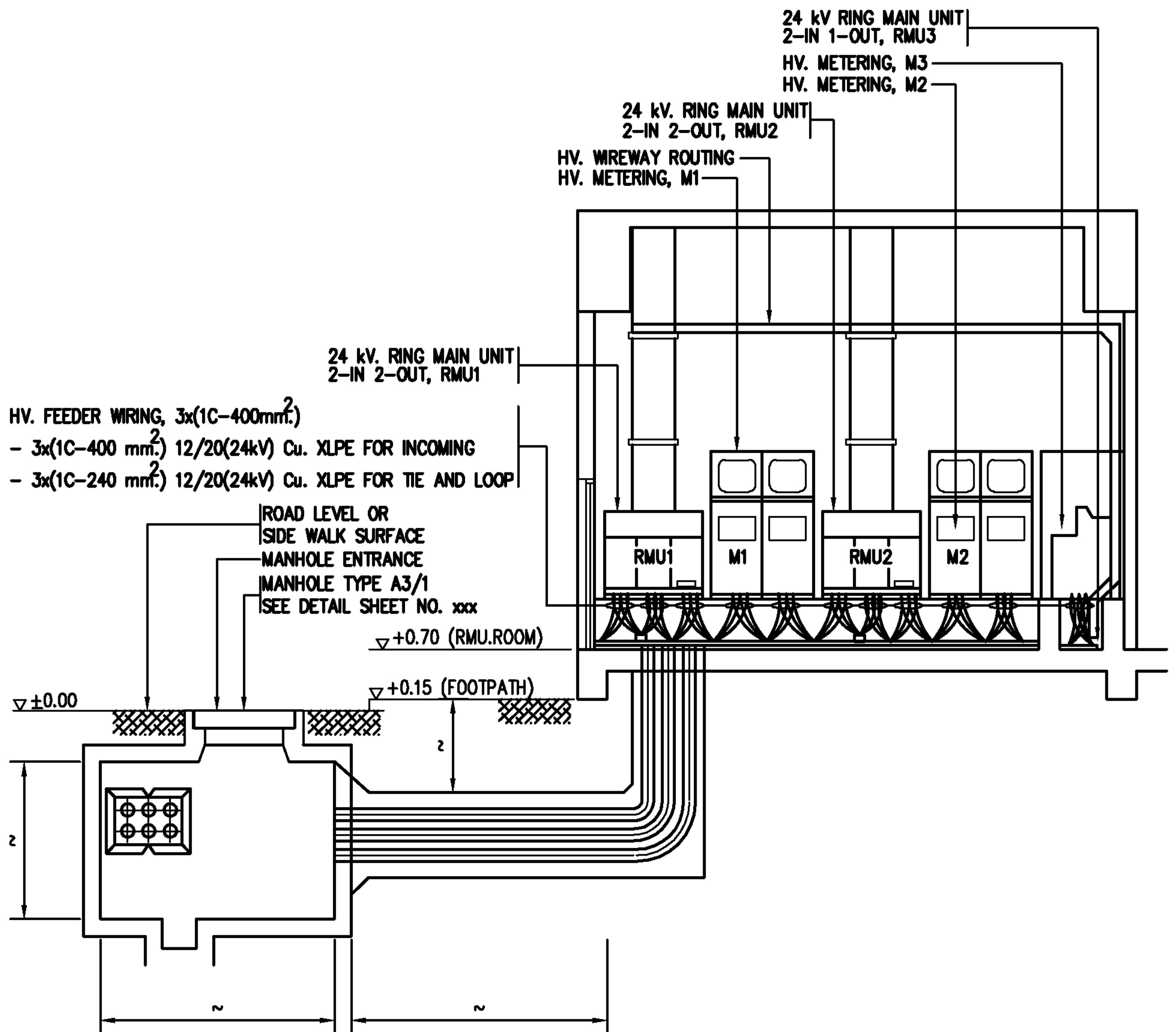
TYPICAL DETAIL MANHOLE TYPE A3/1 และสาย INCOMMING
